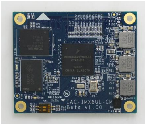
核心板正面
